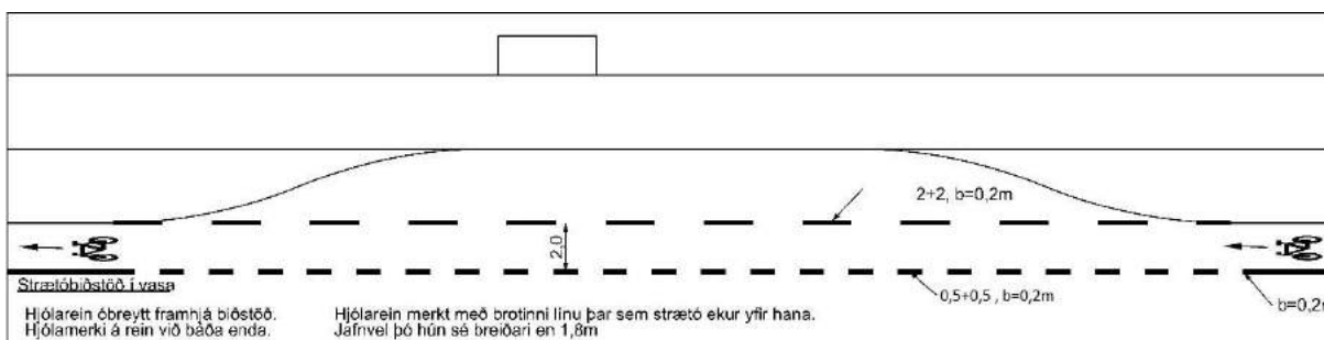
MYND 55 Hjólarrein liggur fram hjá biðstöð í útskoti.
