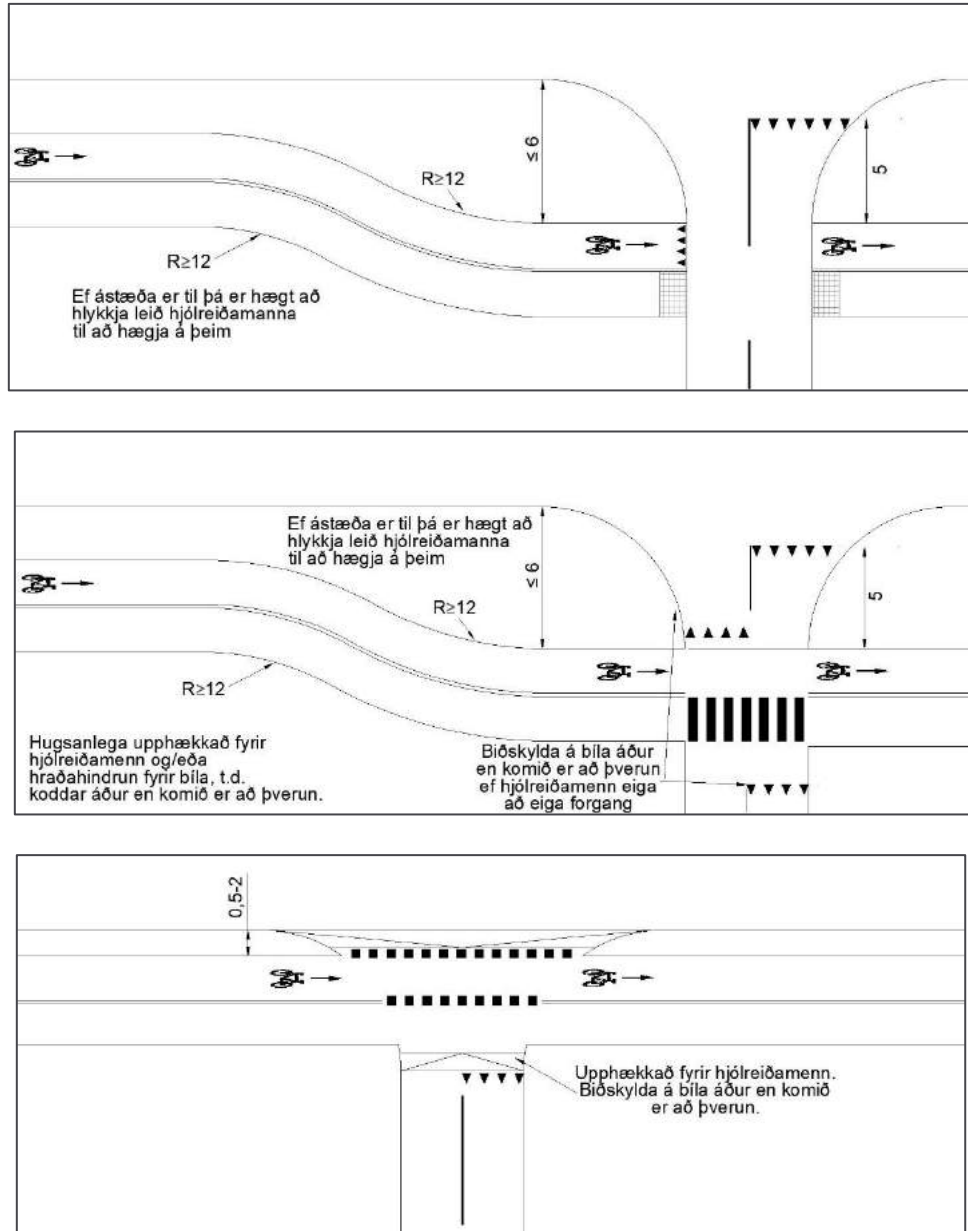
MYND 42 Hjólastígar með einstefnu þverar hliðargötu. Efst: Stígur 6 m frá, hjólríðamenn víkja fyrir akandi. Miðja: Stígur 6 m frá, biðskylða á ökumenn. Neðst: Stígur við götu, biðskylða á ökumenn.
